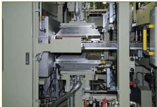
●成形ゾーン
