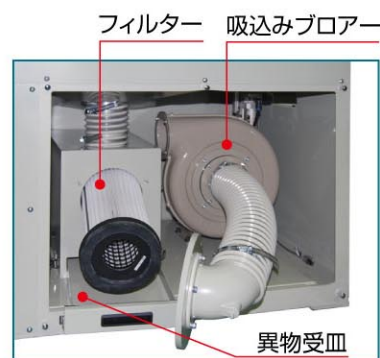
前面扉内部の吸込みブローア及び集塵装置
